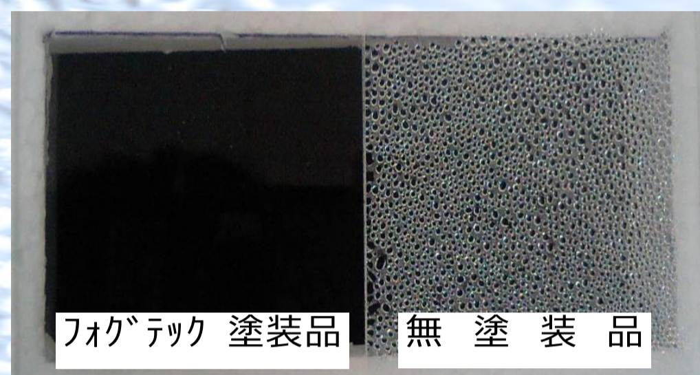
防曇性試験結果 (内面40℃98%RH 外面10℃)
